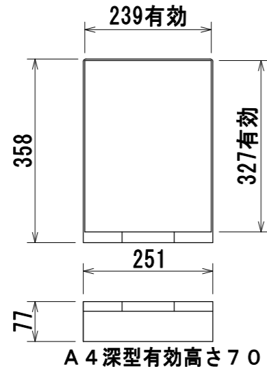
引出詳細図
