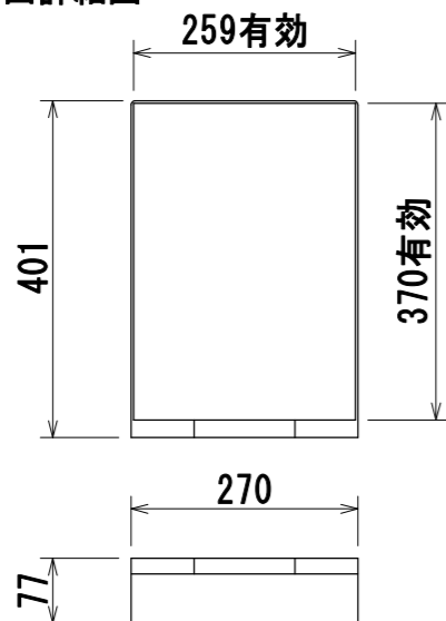
引出詳細図
