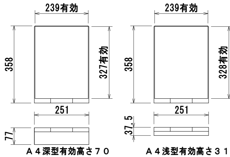
引出詳細図
