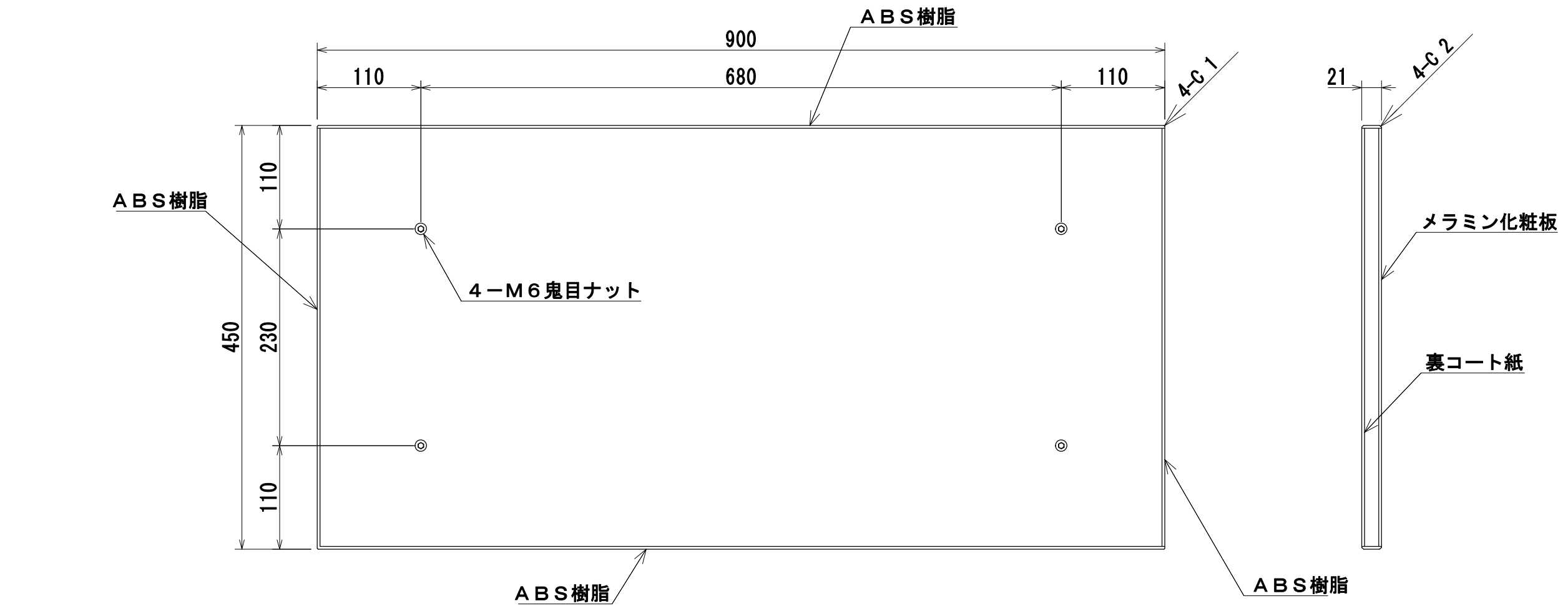
天板断面図 1 / 2
